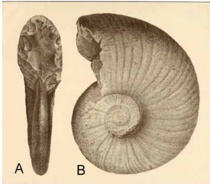
Nálezy amonitů z Poděbrad posloužily i v historické odborné literatuře – vyobrazení Parapuzosia (Austoniceras) austenit z Fričovy publikace z roku 1872.
